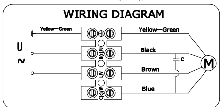
WIRING DIAGRAM (接线图) :
